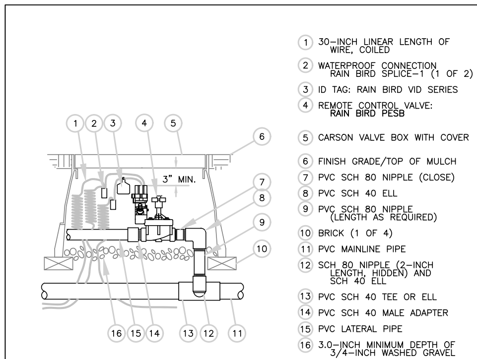
B RAIN BIRD PESB RCV
